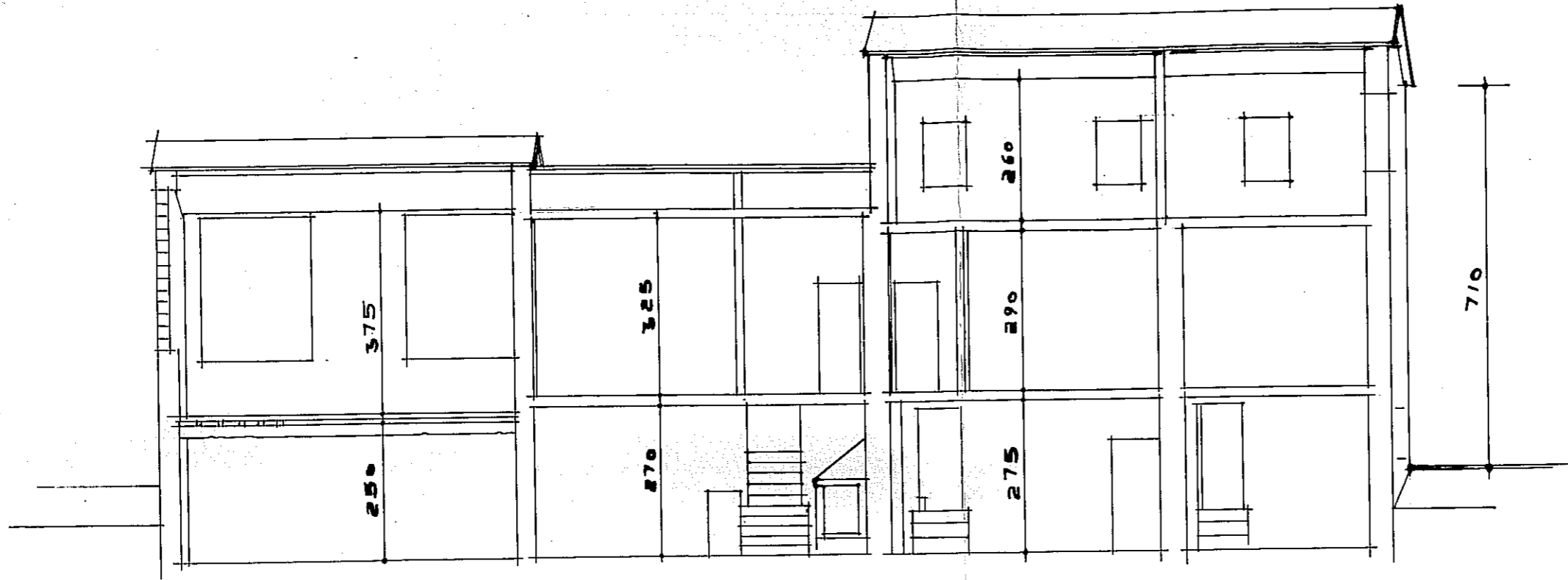
SEZIONE A-A
