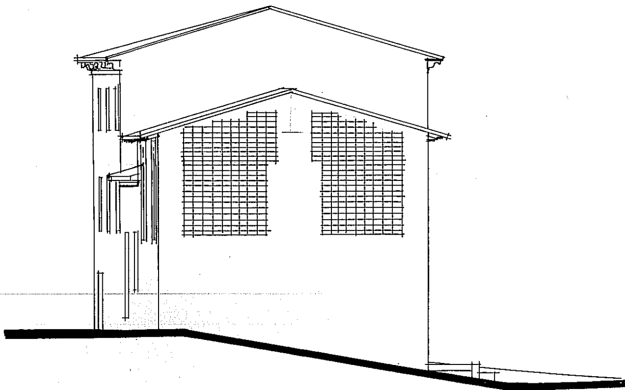
FRONTE OUEST
